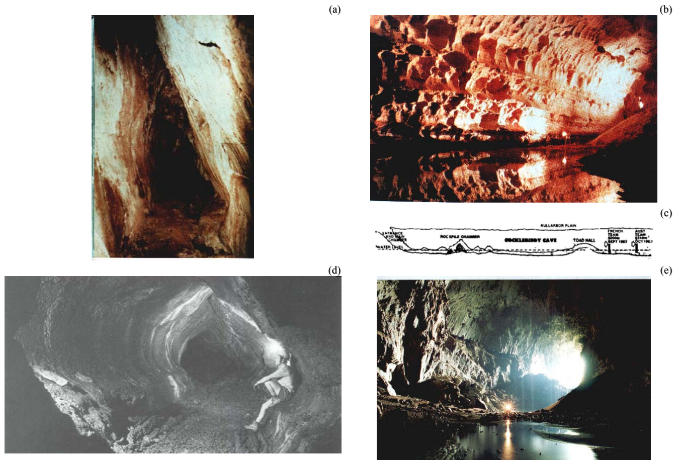
Rys. O6. Gładkie, długie, proste, geometrycznie ukształtowane i namagnesowane tunele wypalane podczas podziemnych przelotów UFO. Pokazane zostały tutaj przykłady już istniejących na Ziemi takich tuneli - po ilustrację zasady ich formowania patrz też rysunek F31.
