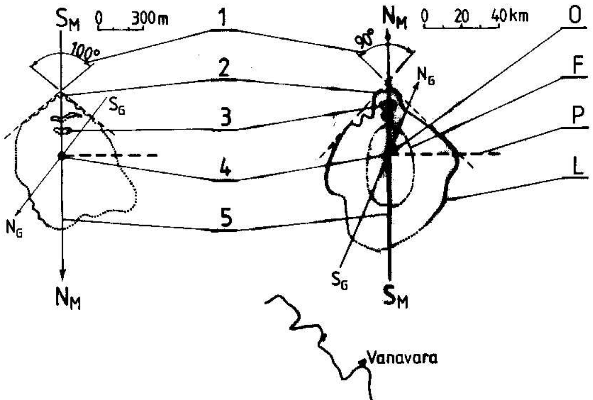
Rys. O5. Porównanie podobieństw występujących pomiędzy konfiguracją krateru Tapanui i obszarem zniszczenia tajgi w miejscu eksplozji tunguskiej. Istnienie takich ścisłych podobieństw świadczy że pochodzenie obu tych miejsc jest analogiczne, tj. z potężnych eksplozji napowietrznych. Najbardziej widoczne zgodności obu miejsc dotyczą: (1) związku pomiędzy kątem wejścia fal uderzeniowych, a odległością miejsca eksplozji od najbliższego bieguna magnetycznego (to z kolei posiada związek z kątem nachylenia eksplodującego cygara UFO), (2) kształcie obszaru wejściowego fal uderzeniowych, (3) nieregularnym zniszczeniu w miejscach załamywania się fal uderzeniowych (w miejscach tych drzewa tajgi ułożone są "wichrowato", natomiast w kraterze Tapanui występują wydymowate nasypiska gruntu), (4) położenia środka eksplozji "O", (5) zorientowania osi zniszczenia wzdłuż południka magnetycznego, itp. Oznaczenia: S_G/NG - kierunki geograficzne; S_M/NM - kierunki magnetyczne, które pokrywają się z przebiegiem głównych osi zniszczenia.
